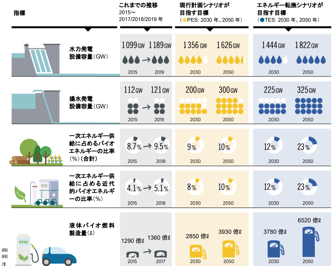
図 S.5 どのような未来のエネルギーシステムにも不可欠：水力とバイオエネルギー 水力発電設備容量、バイオエネルギーの比率、液体バイオ燃料の製造
