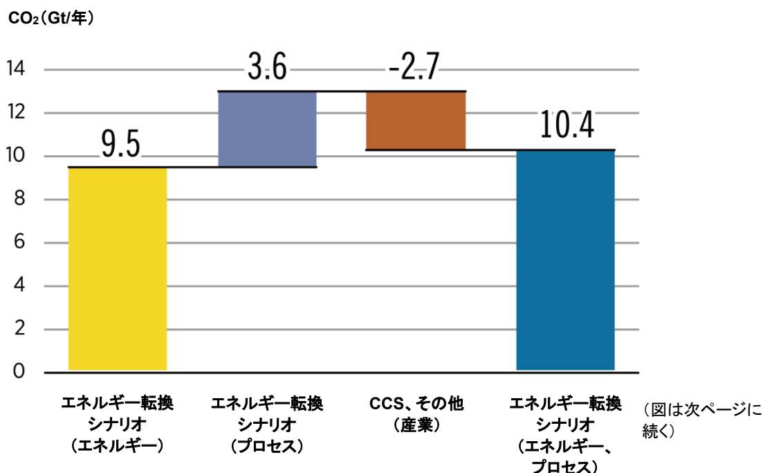
図 5.2 脱炭素深化見通し： ネットゼロ、さらに最終的にゼロカーボンの達成（図は次ページに続く） エネルギー転換シナリオで残存するエネルギーおよび産業プロセス関連の CO 2 排出量
