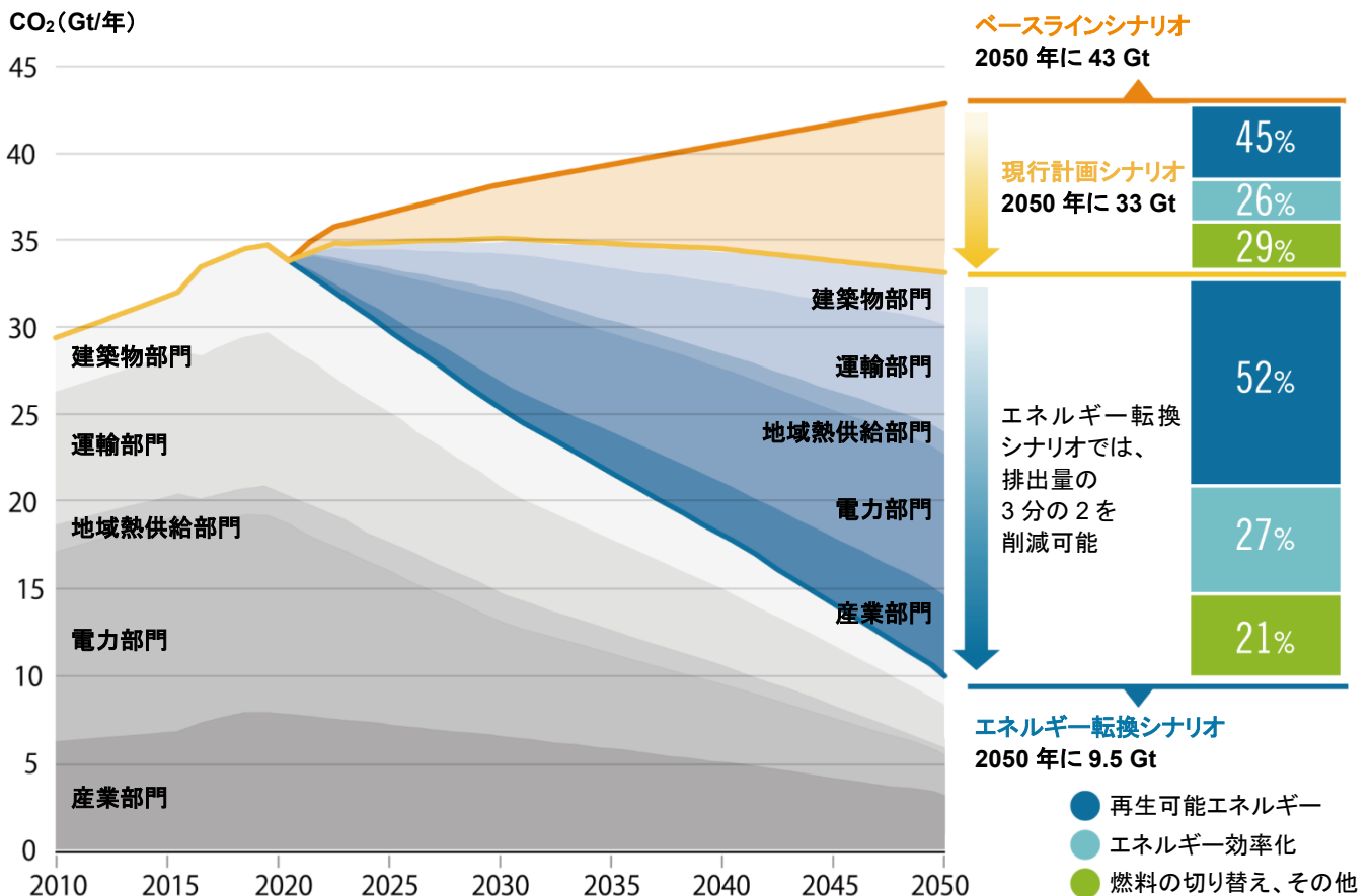
図 S.7 排出量削減の大部分：再生可能エネルギーとエネルギー効率化
