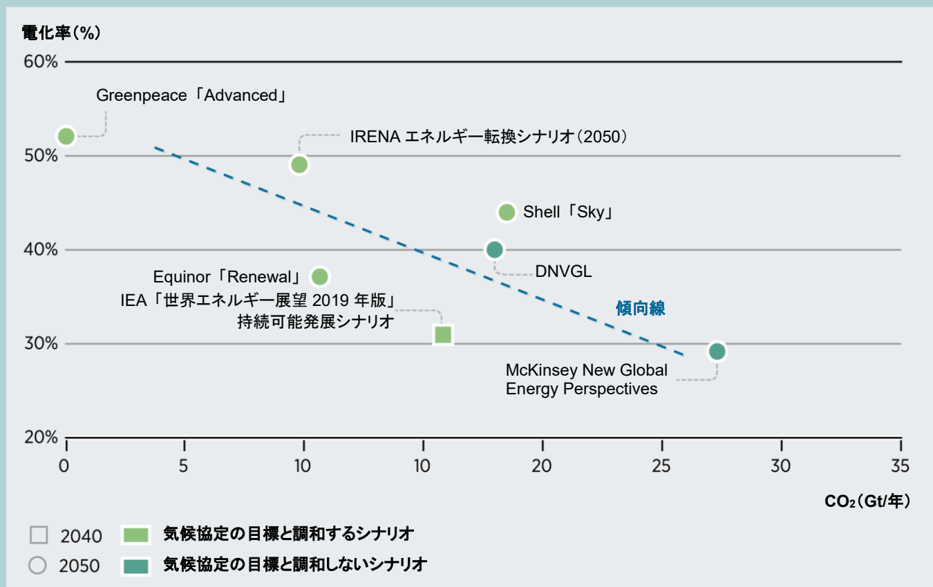
図 1.16 未来に対するさまざまなビジョン：他の主なエネルギー研究で提示されたシナリオ さまざまなエネルギーシナリオにおける、2050年の世界のエネルギー関連のCO 2 排出量と電化率
