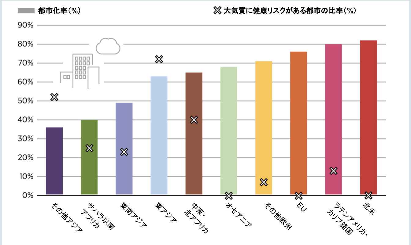
図 3.7 都市の大気質：急成長する都市の大きな懸念事項 都市化と都市大気質
