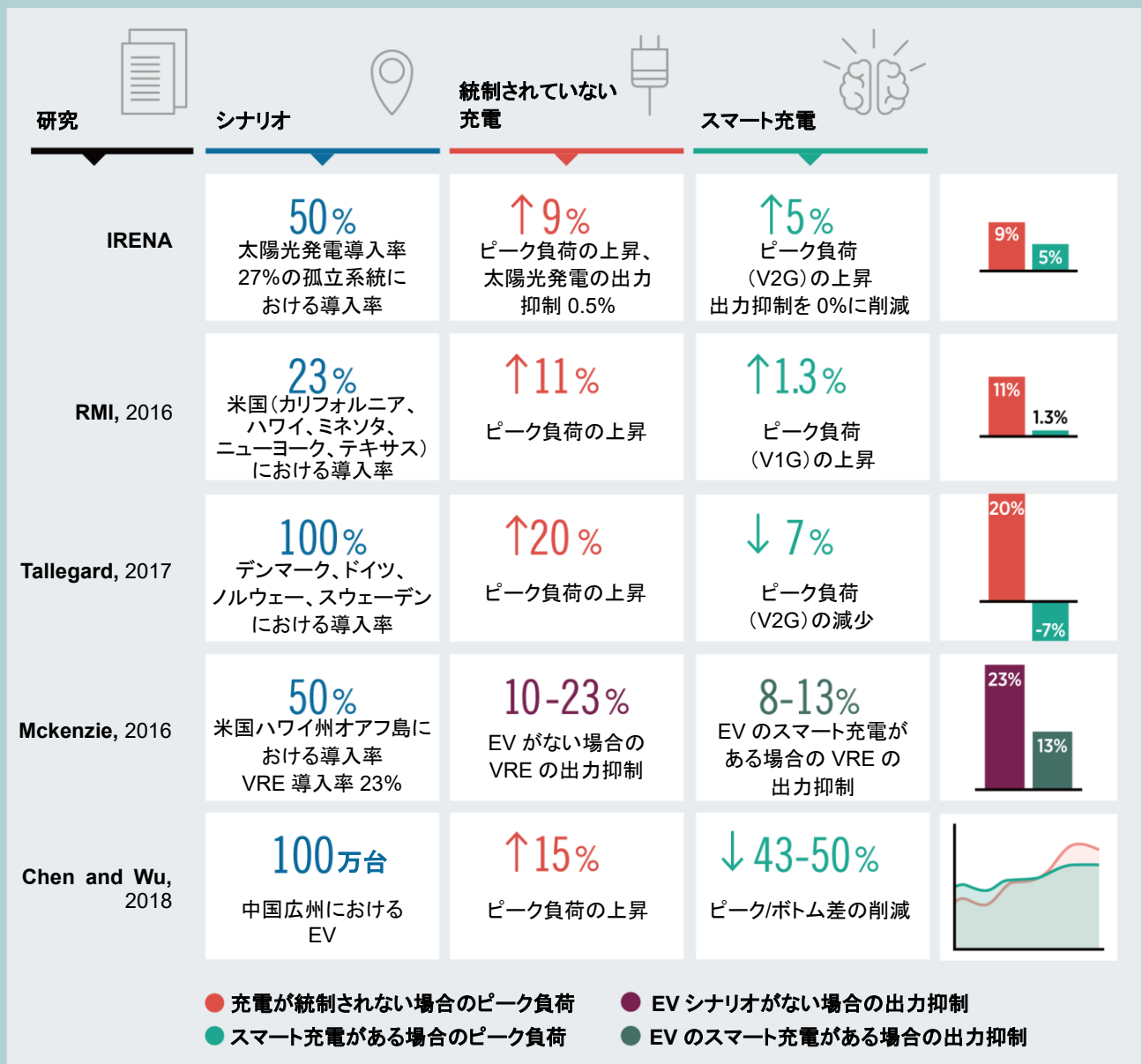
図 1.13 EV のスマート充電を実現する技術、ビジネスモデル、規制の枠組み EV のスマート充電が電力系統に及ぼす影響
