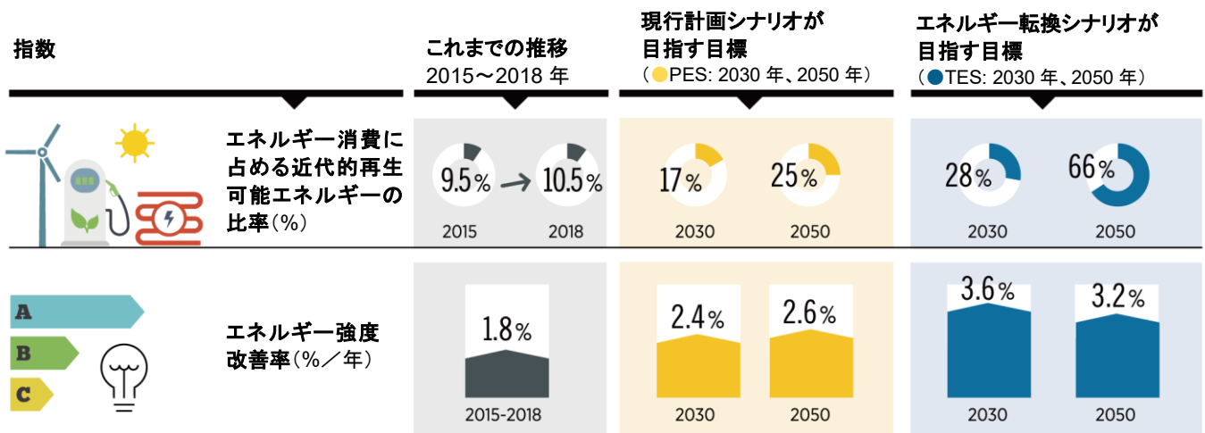
図 S.2 世界のエネルギーミックスに占める再生可能エネルギーの比率：6 倍への増加が必要 再生可能エネルギーの導入率とエネルギー効率改善度
