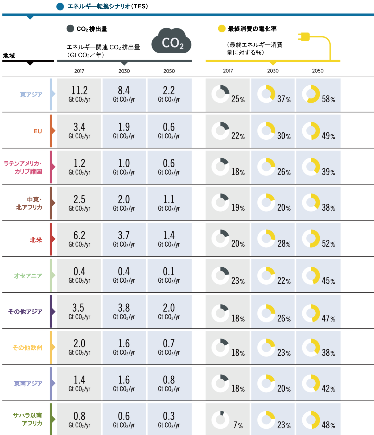
図 3.10 世界のエネルギー脱炭素化：地域ごとに異なるエネルギー転換への道筋 エネルギー転換シナリオにおける CO 2 排出量、電化率などの地域別指数
