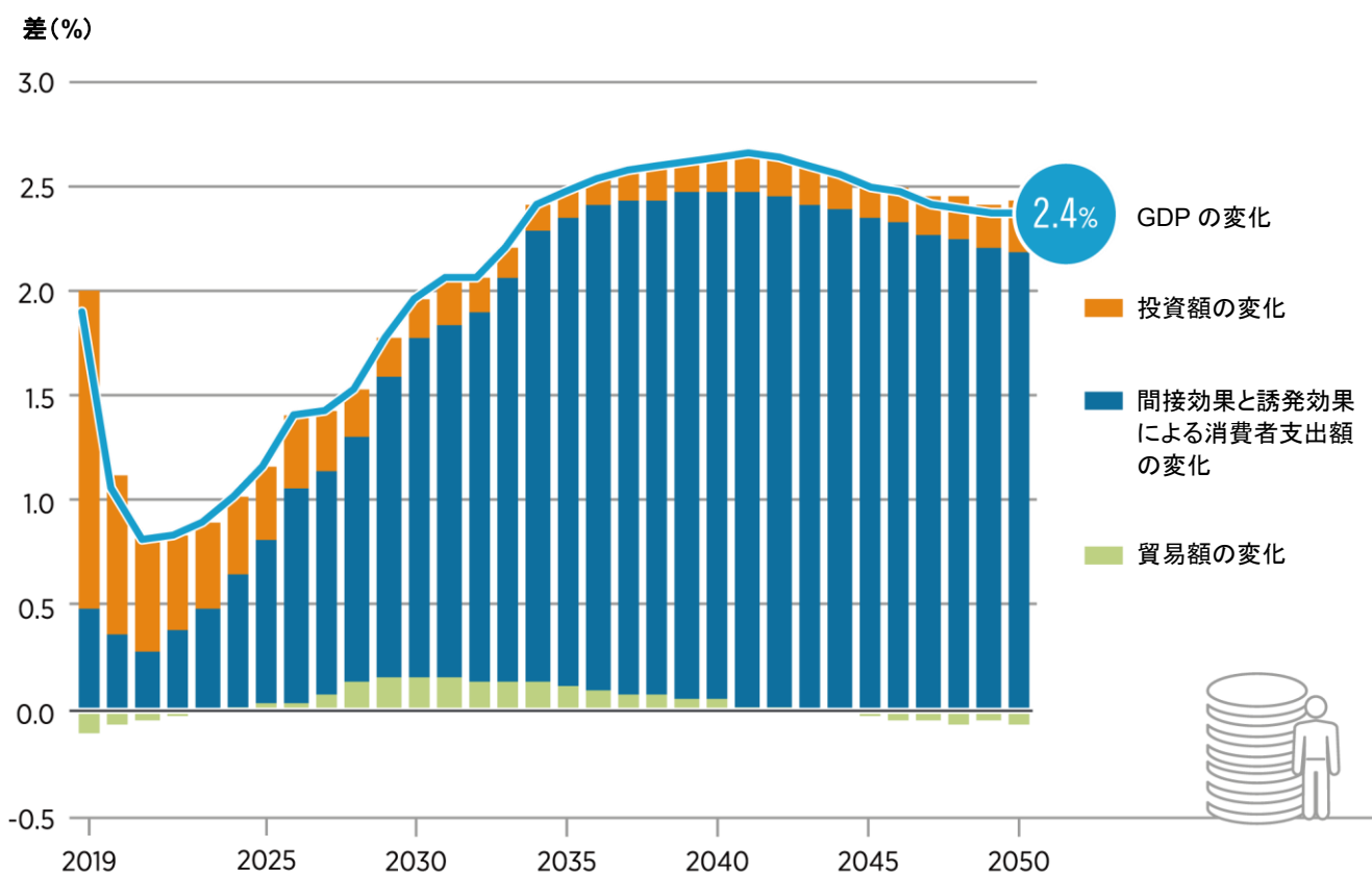
図 2.8 エネルギー転換シナリオは世界の GDP を後押し
