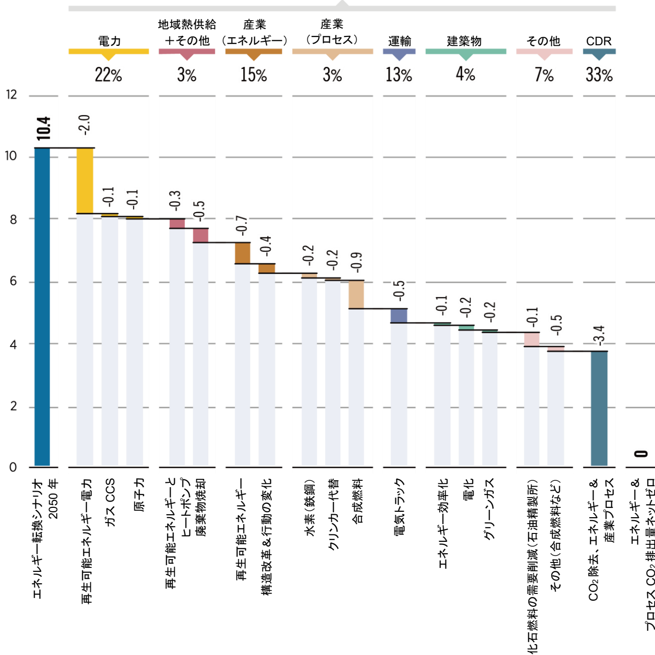
遅くとも 2060 年までにエネルギーおよびプロセス部門をネットゼロにするための脱炭素深化見通し(Gt CO 2 ) 削減の部門別内訳(エネルギー転換シナリオからネットゼロへ)
