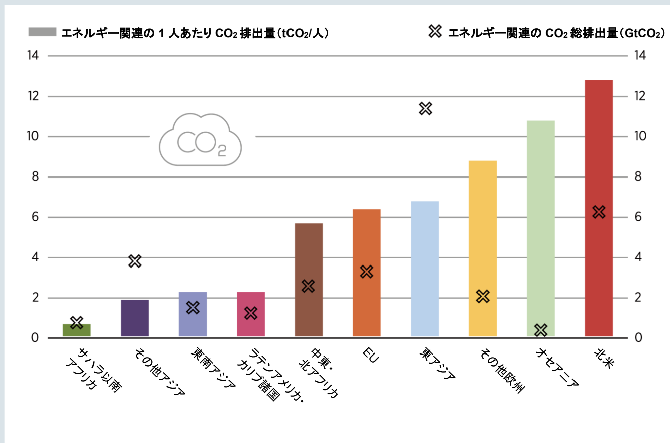
図 3.4 エネルギー関連の CO 2 排出量: 各地域の現行水準
